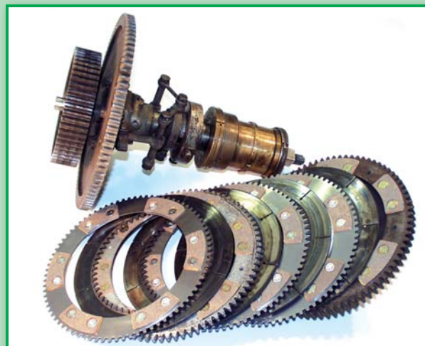
BUGATTI 46 2T r.v.1929 - před kompletací
